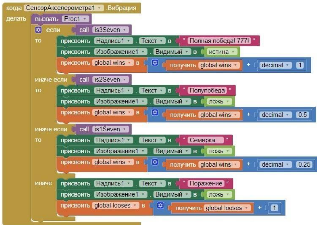
Рисунок 197. Программные блоки, выполняемые при встряхивании мобильного устройства
