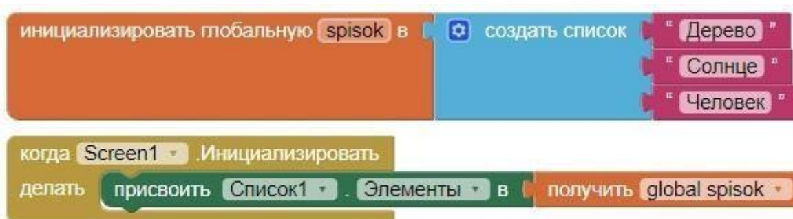
Рисунок 234. Инициализация компоненты Список1
