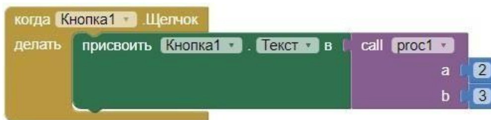
Рисунок 83. Пример использования блока вызова процедуры
