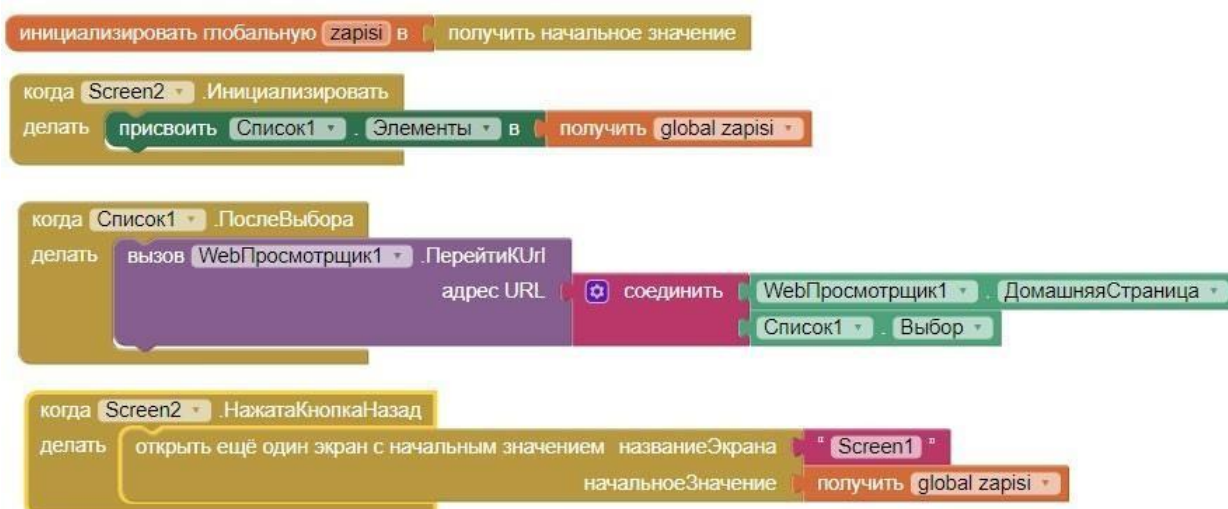
Рисунок 251. Общая схема блоков экрана Screen2
