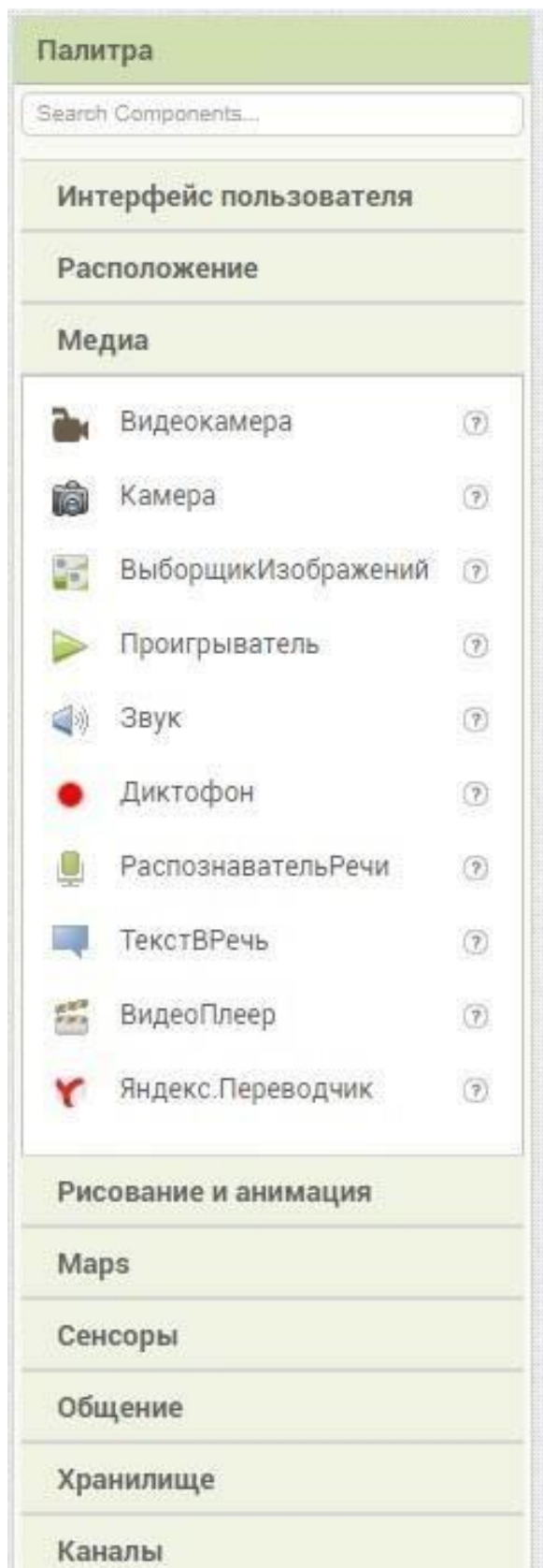
Рисунок 38. Функционал «Медиа»
