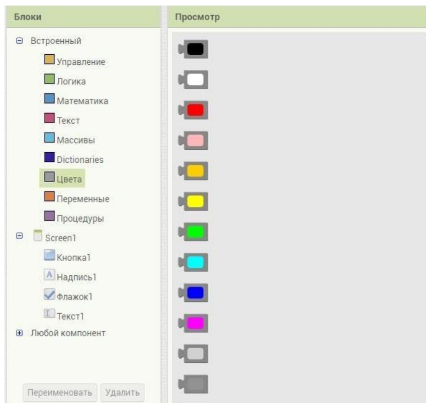
Рисунок 61. Выбор цвета
