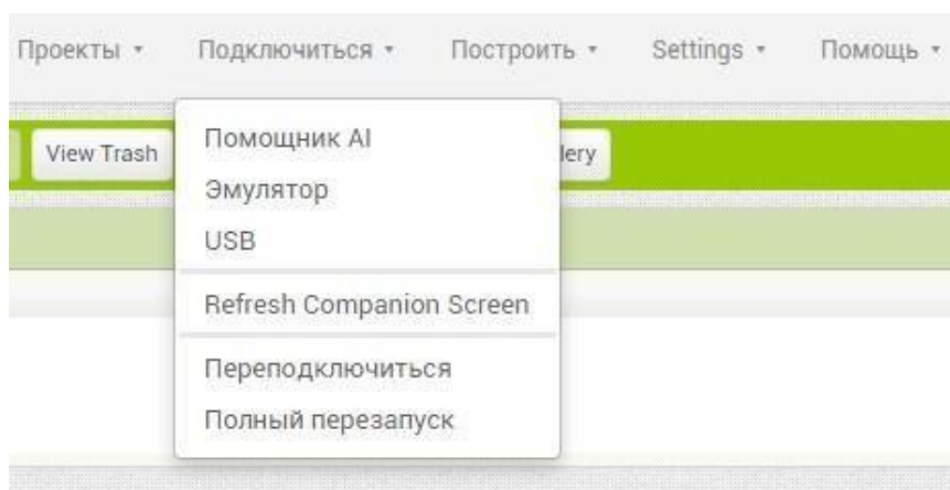
Рисунок 27. Меню «Подключиться»
