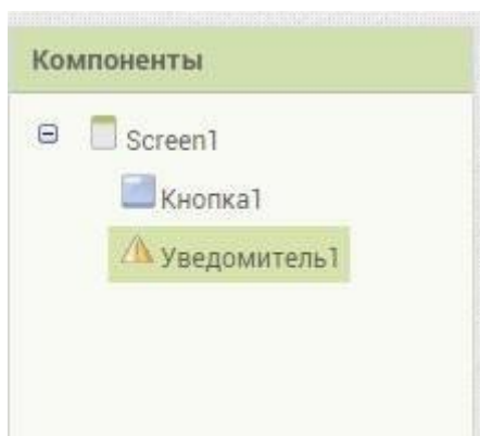
Рисунок 90. Схема компонент
