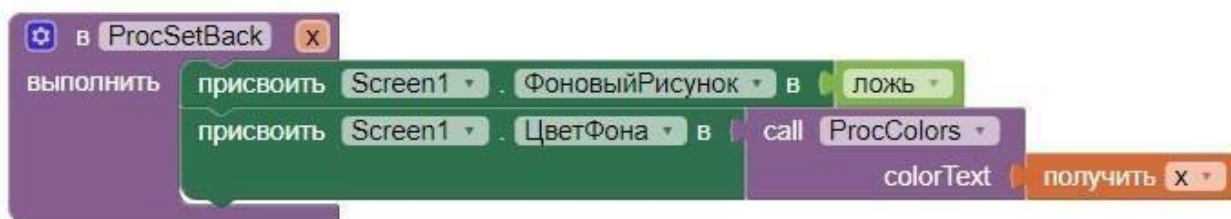
Рисунок 172. Процедура ProcSetBack
