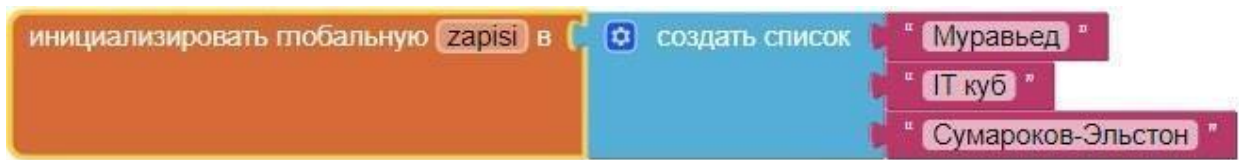
Рисунок 222. Инициализация массива
