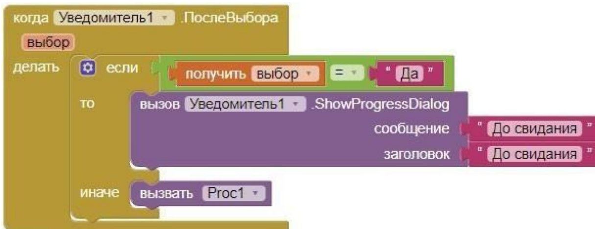
Рисунок 215. Обработчик выбора кнопок уведомления
