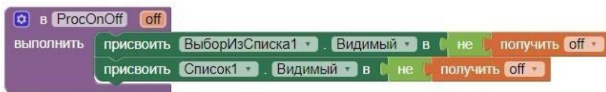
Рисунок 173. Процедура ProcOnOff
