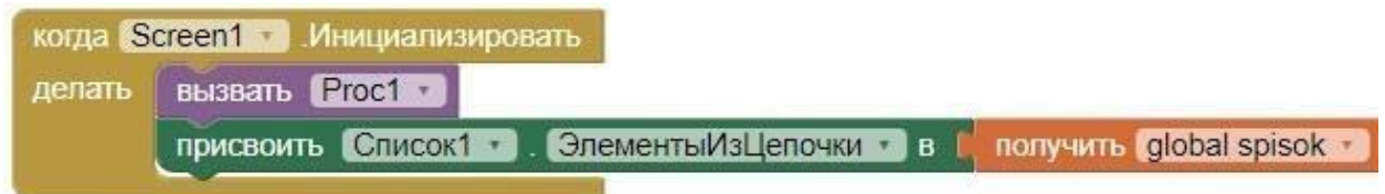
Рисунок 264. Инициализация экрана
