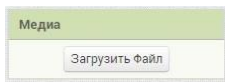
Рисунок 180. Загрузка медиафайлов
