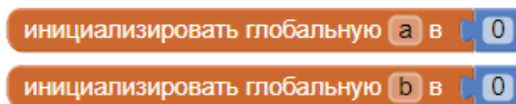
Рисунок 123. Инициализация переменных
