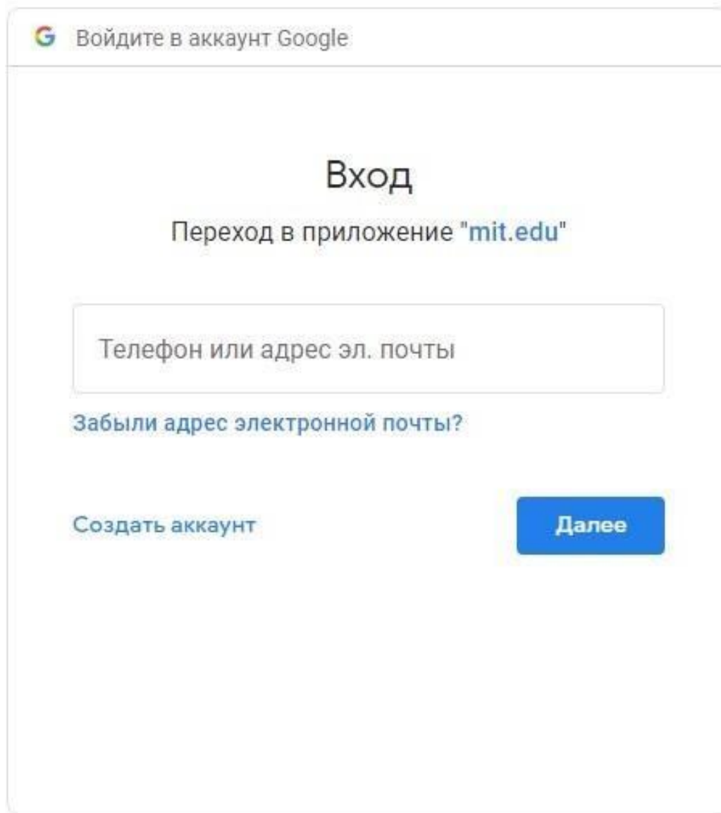
Рисунок 15. Ввод логина
