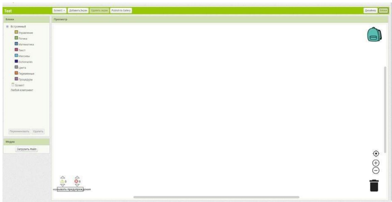
Рисунок 47. Окно «Блоков»
