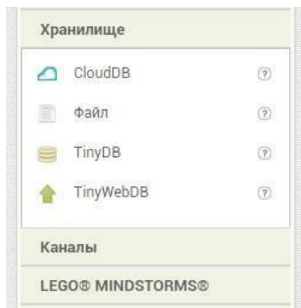
Рисунок 43. Функционал «Хранилище»
