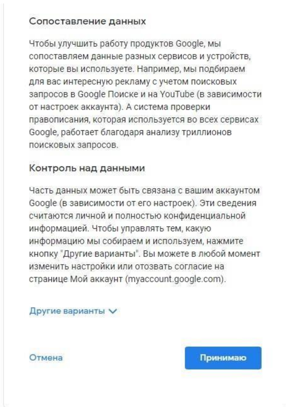
Рисунок 12. Подтверждение договора
