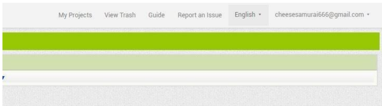
Рисунок 19. Выбор языка
