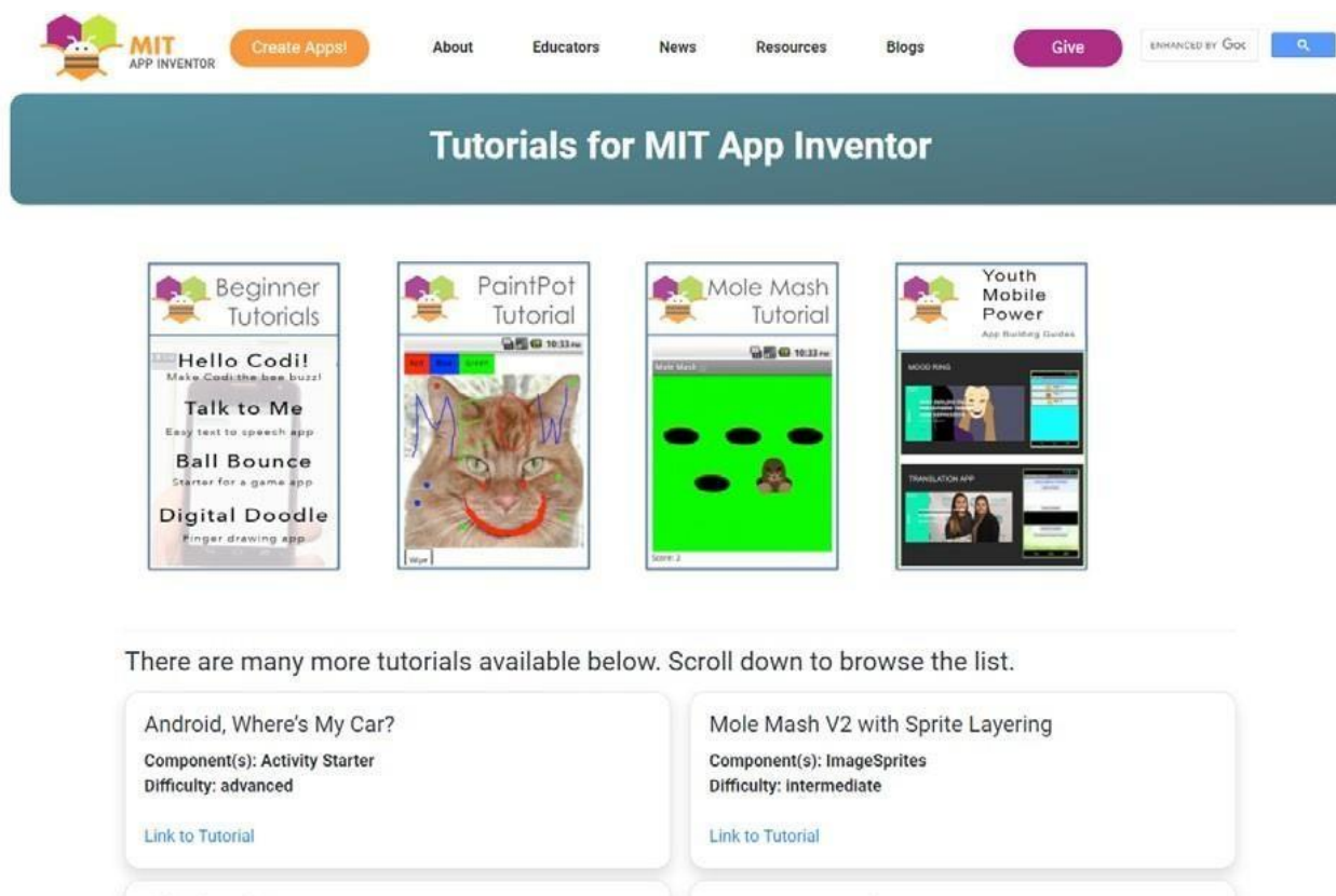
Рисунок 32. Функционал «Уроки»
